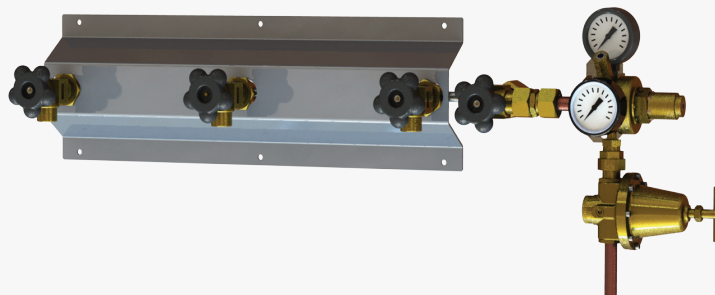
Manifold económico con válvula principal de cierre de alta presión opcional
